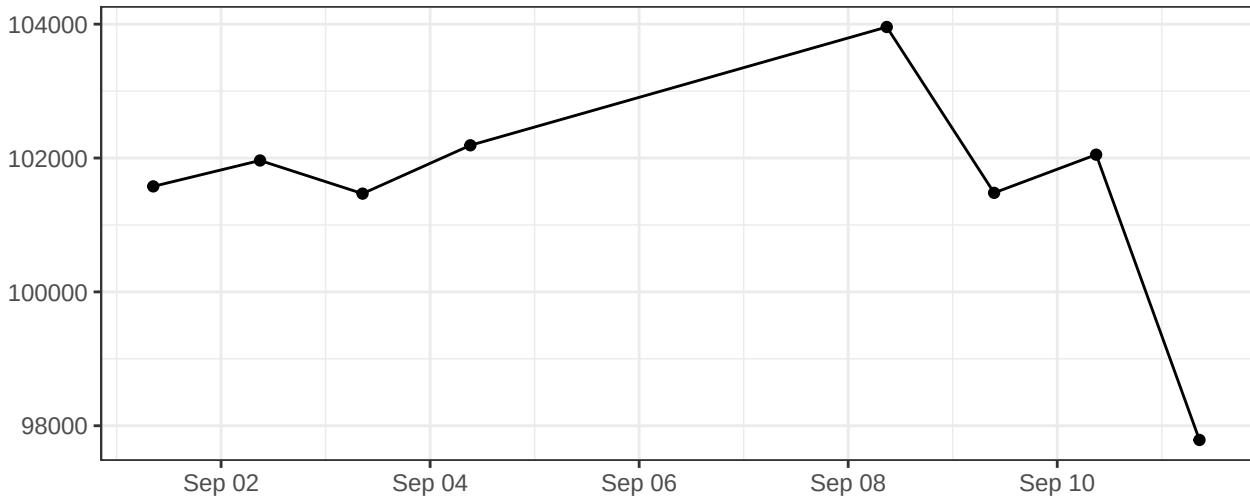
SSC-A
