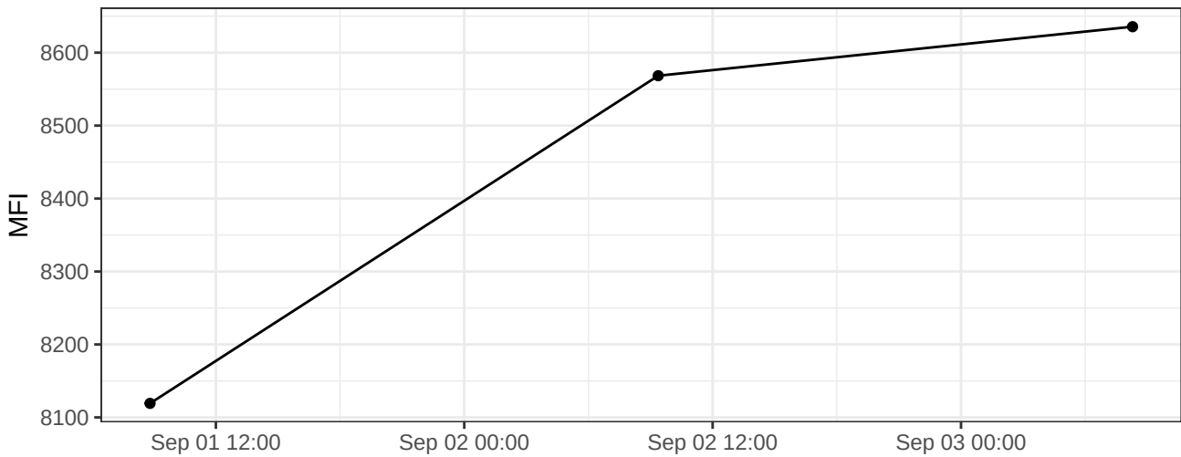
BUV563-A
