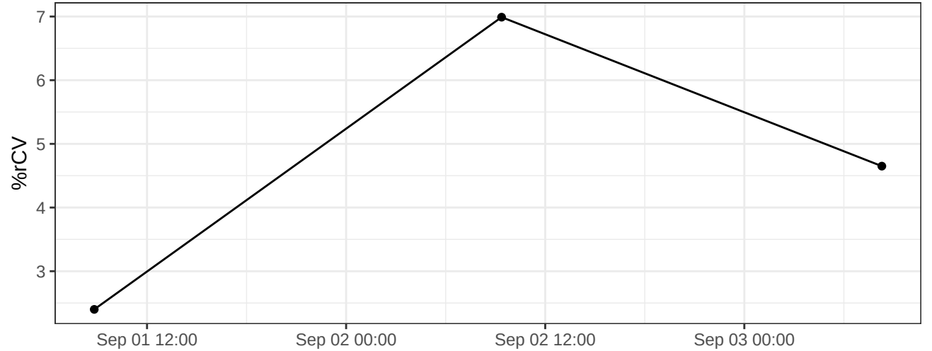
BV711-A-% rCV
