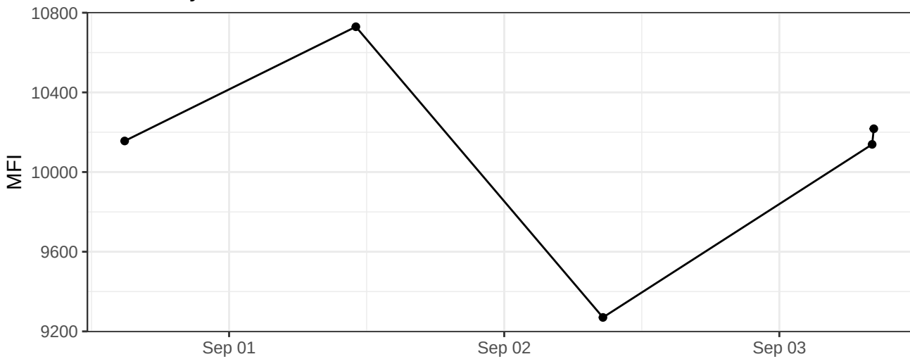
BB790-A
