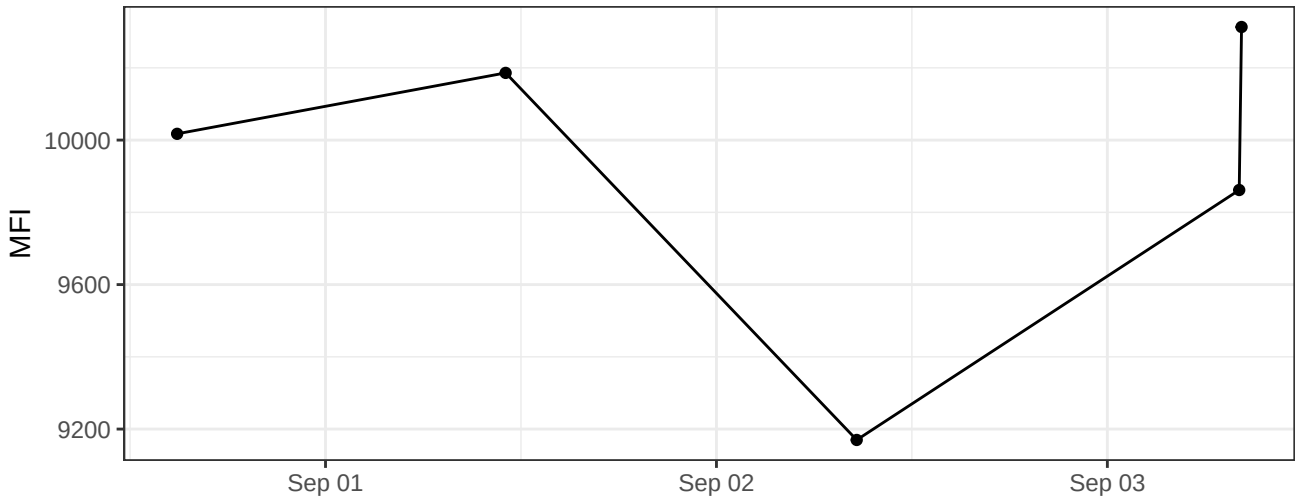
DAPI-A
