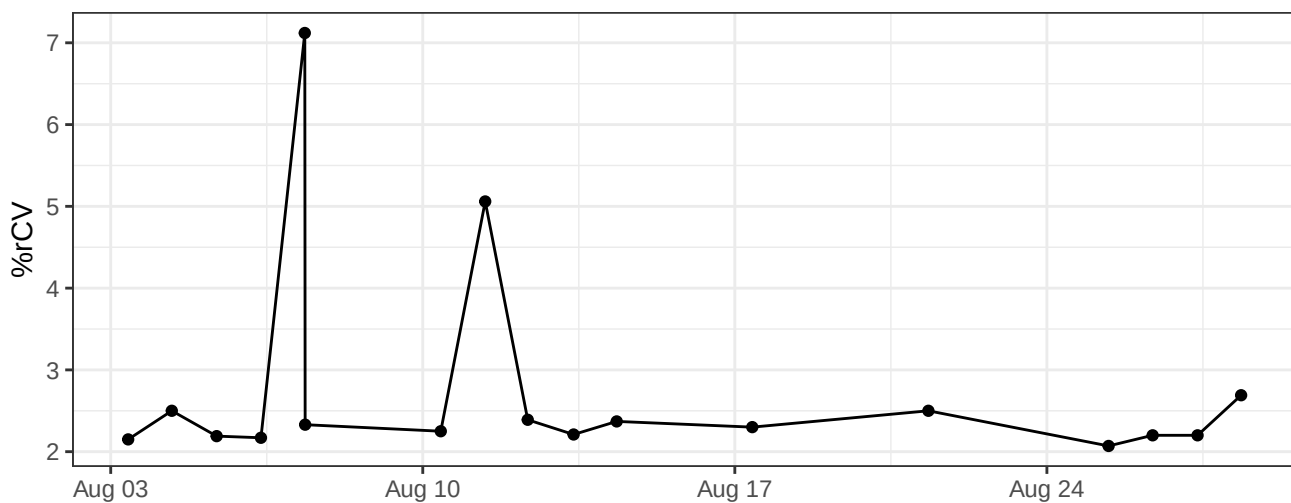
BYG584-A-% rCV
