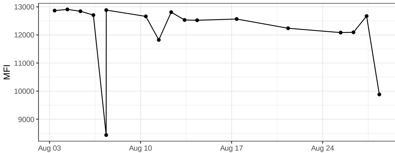
APC-R700-A
