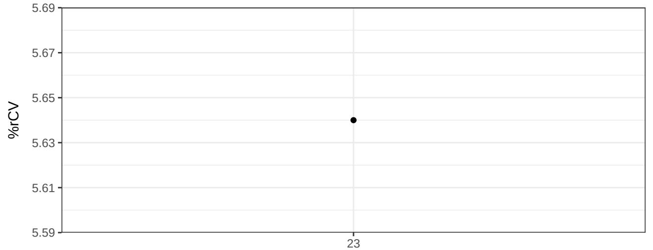
BUV496-A-% rCV
