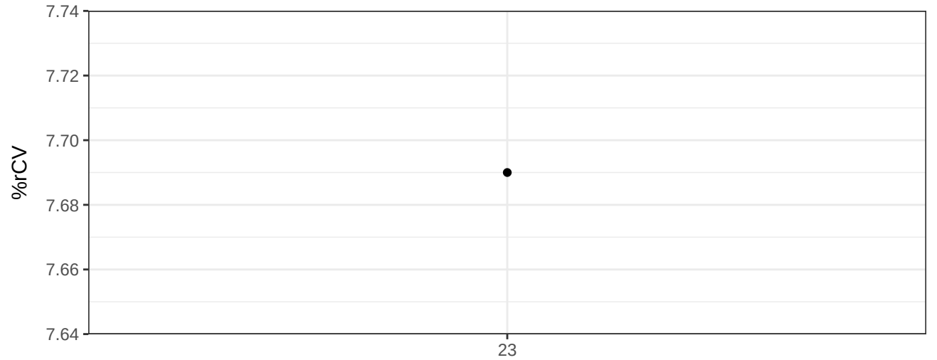
DAPI-A-% rCV
