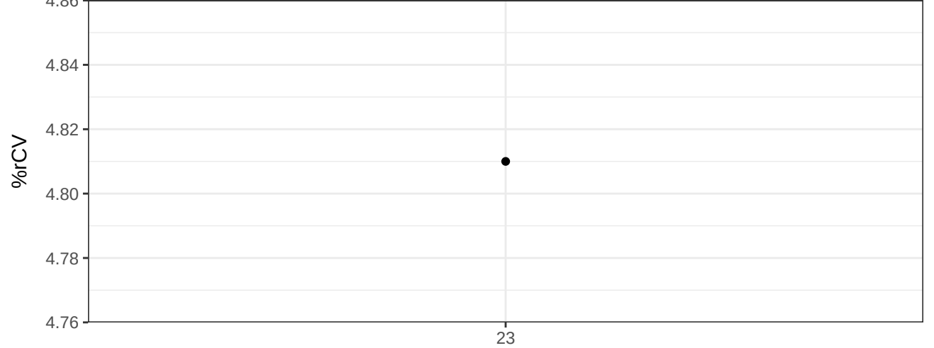
BV510-A-% rCV
