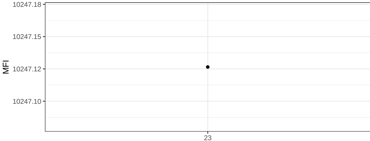
BV786-A
