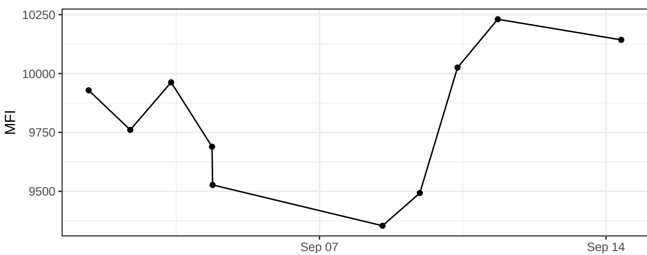
BV786-A
