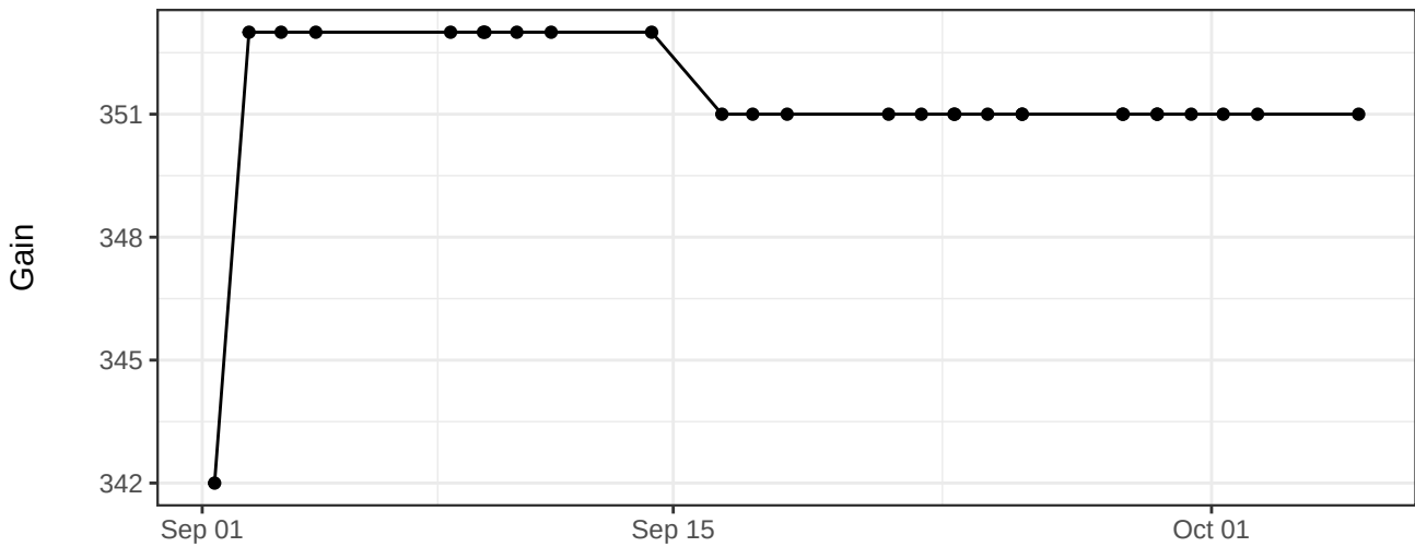
BUV563-A_Gain
