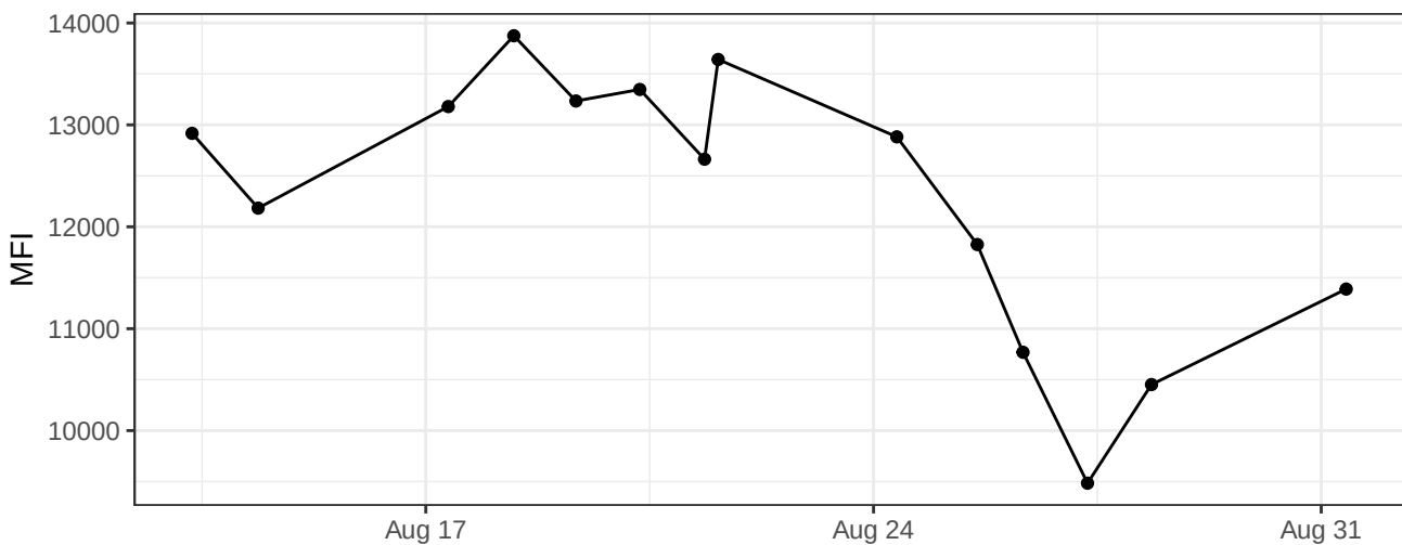
BV510-A
