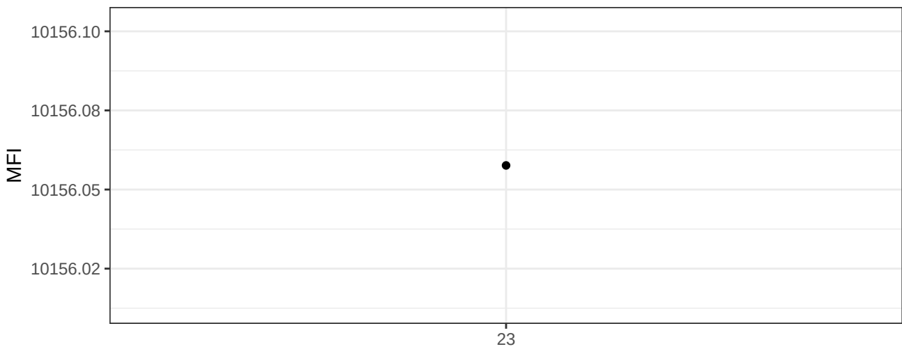
BB790-A
