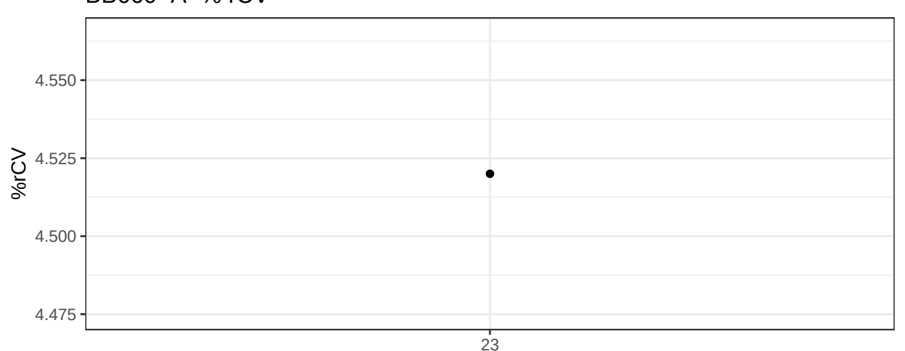
BB660-A-% rCV
