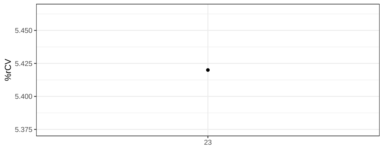
BUV496-A-% rCV
