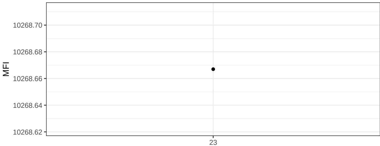
BV750-A
