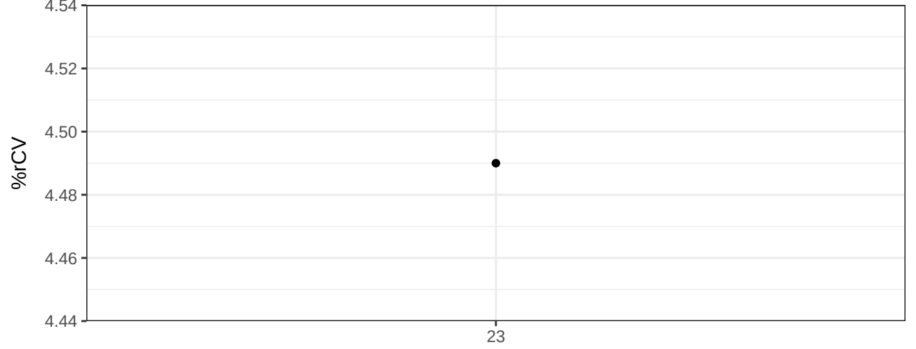
BV650-A-% rCV
