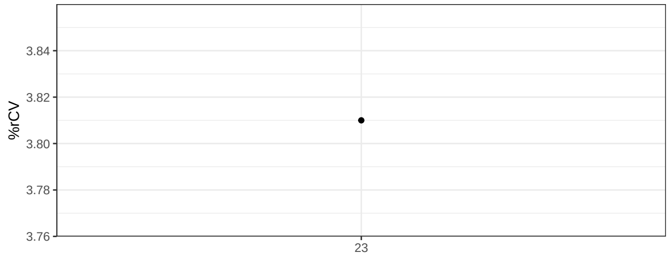
BV750-A-% rCV
