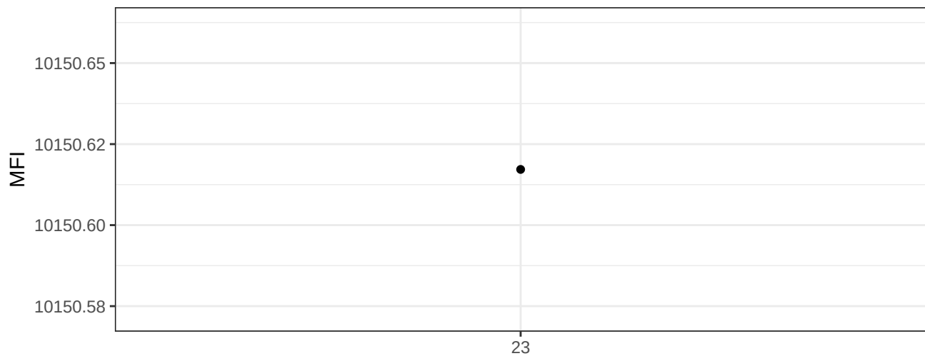
BUV661-A
