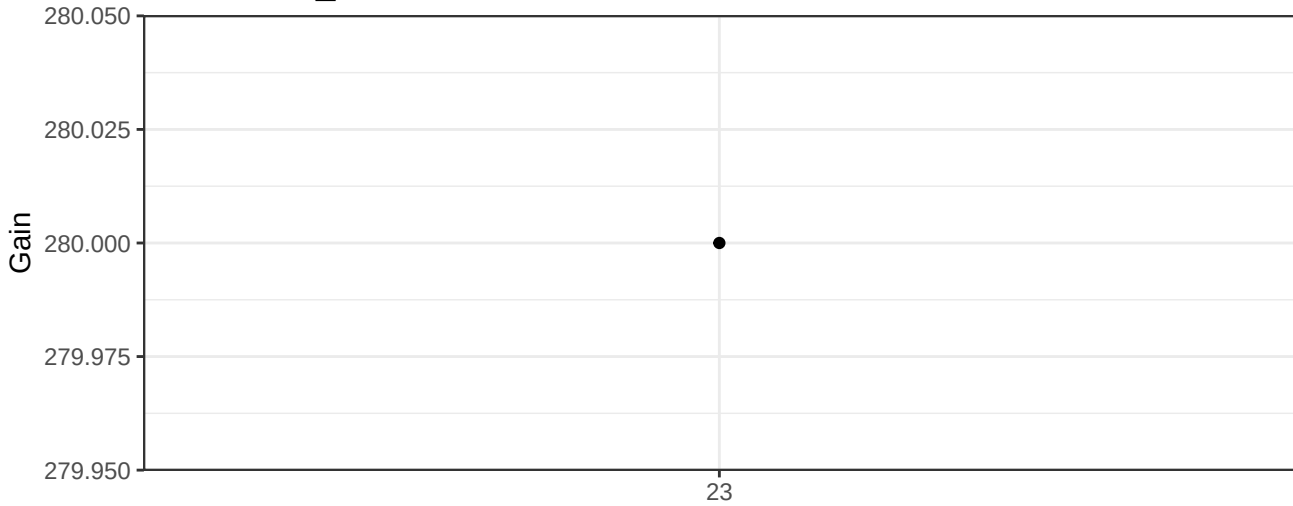
BUV737-A_Gain
