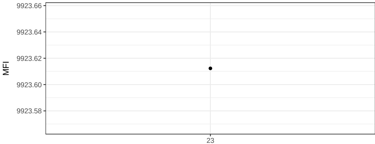
BV786-A
