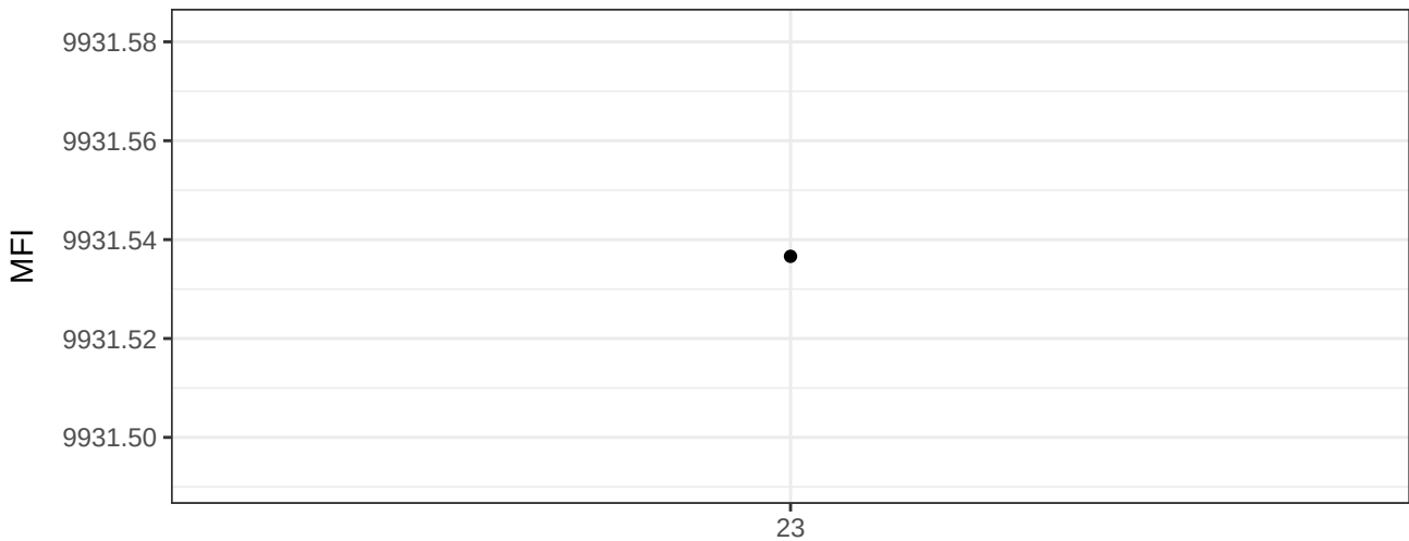
BV421-A
