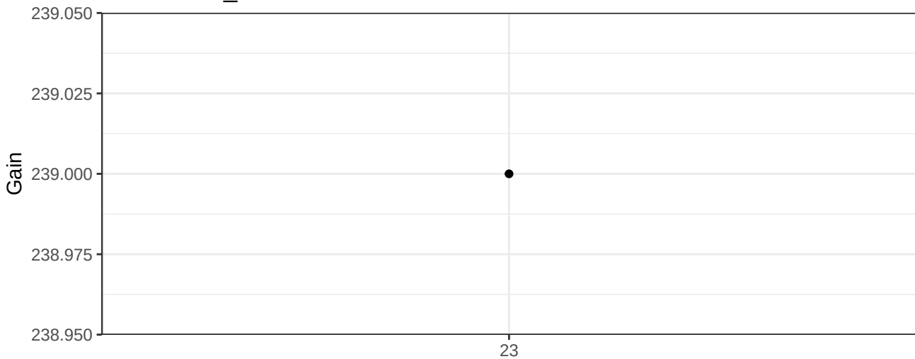
BUV661-A_Gain
