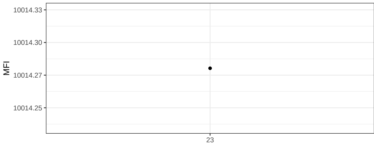
APC-A
