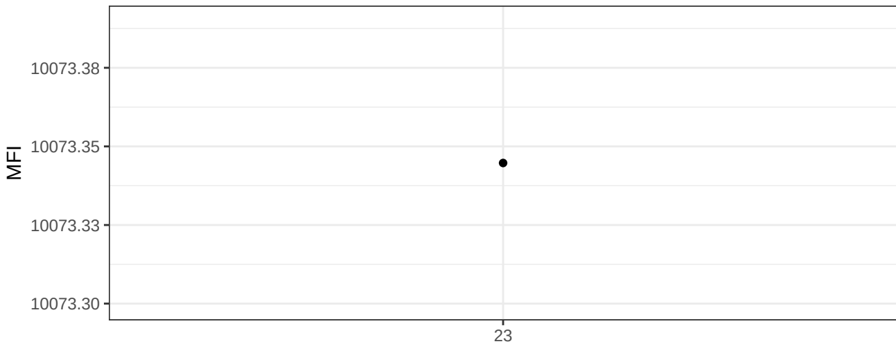
BV605-A
