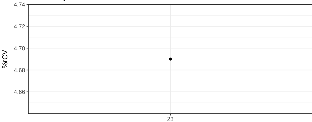
BB790-A-% rCV
