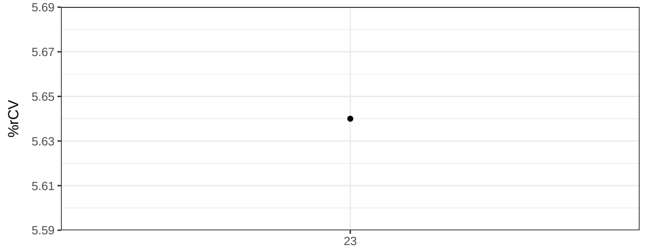
DAPI-A-% rCV
