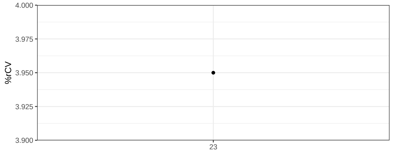
BB630-A-% rCV
