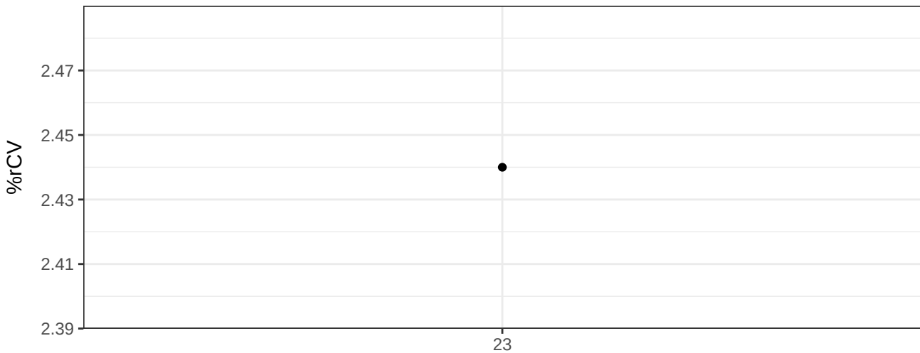
PE-Cy5-A-% rCV
