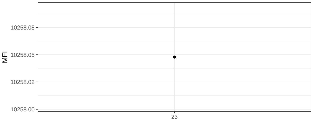
BB660-A
