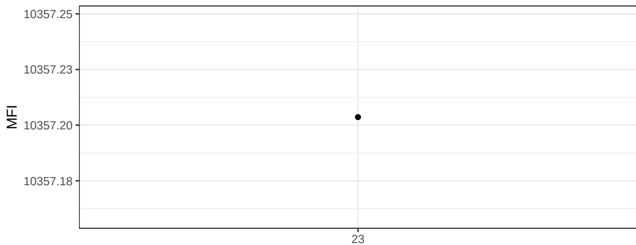
BUV737-A
