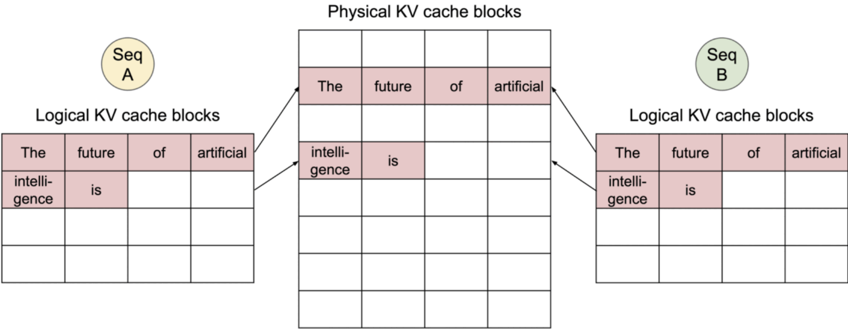
圖片由使用者提供，出自 vLLM PagedAttention 發表文。動畫展示兩個共用同一段 prompt 的 request，如何對應到相同的 physical KV block。
