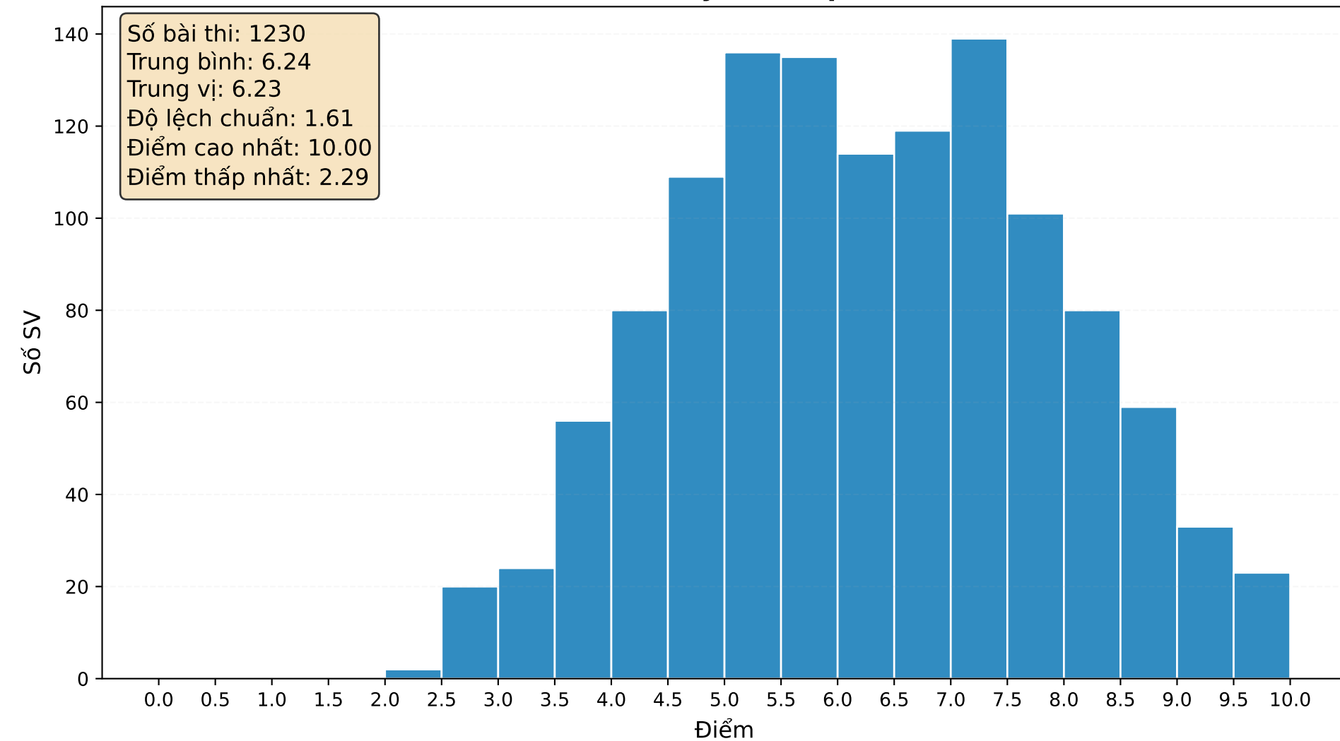
Phổ điểm cuối kỳ toàn bộ sinh viên
