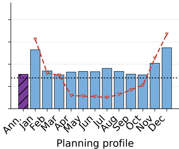
(b) 3x solar
