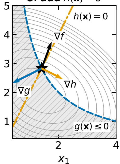
3. add h(\mathbf{x}) = 0
