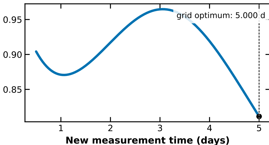
A: minimize trace inverse
