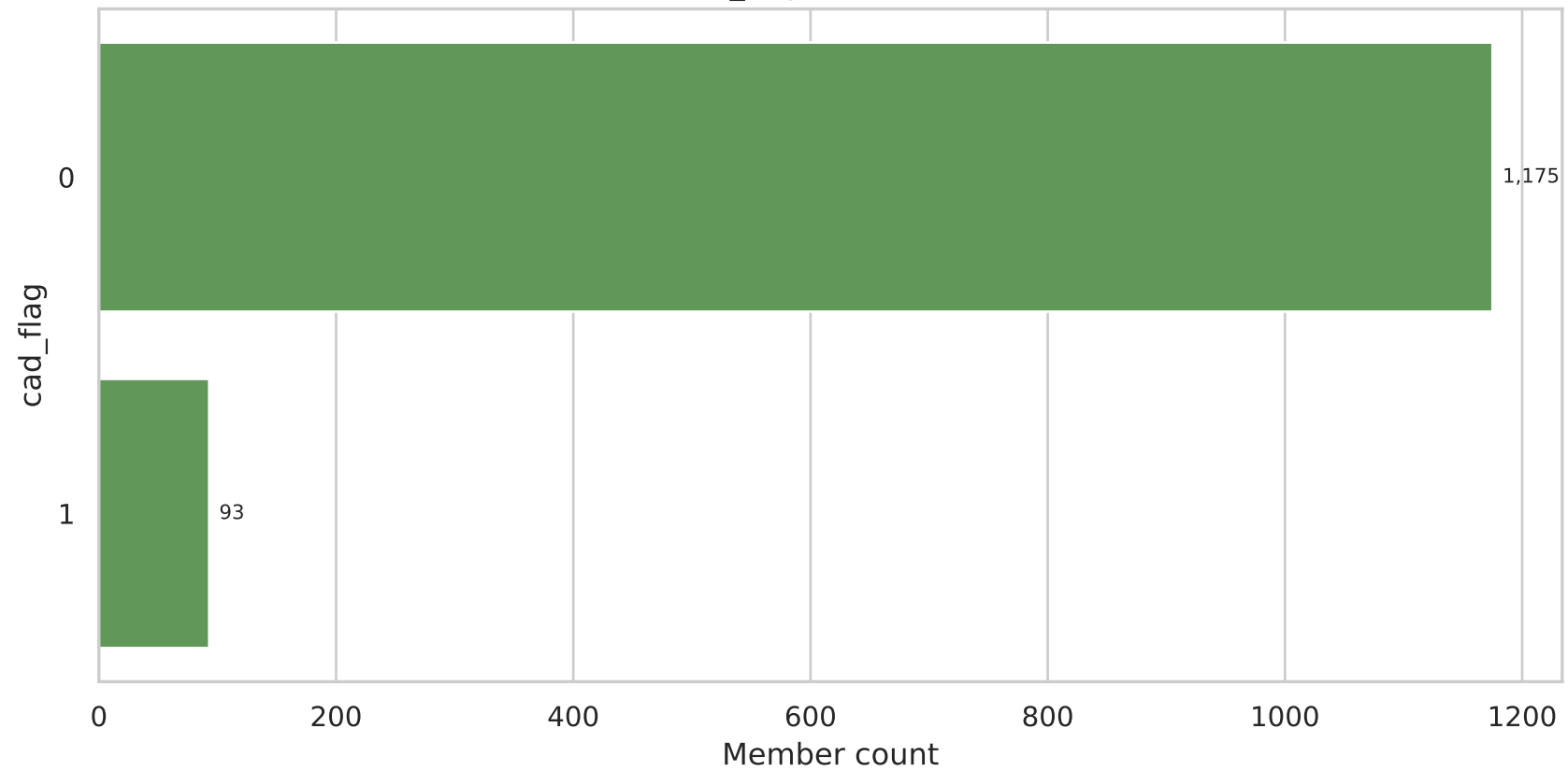
cad_flag Distribution
