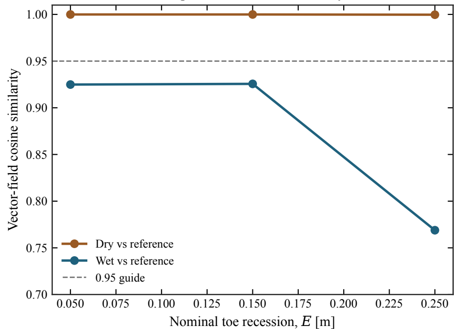
Displacement-mode similarity
