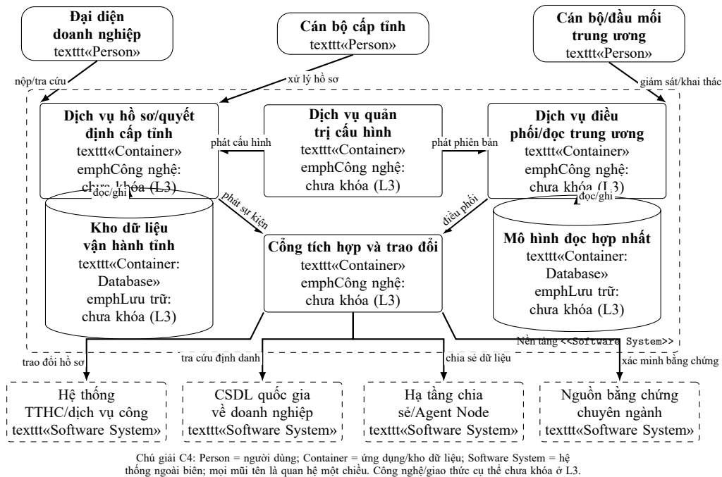
Hình 5. Cấu trúc vùng chứa và ranh giới trách nhiệm – góc nhìn vùng chứa logic dùng các phần tử C4; công nghệ/giao thức cụ thể được giữ ở L3
