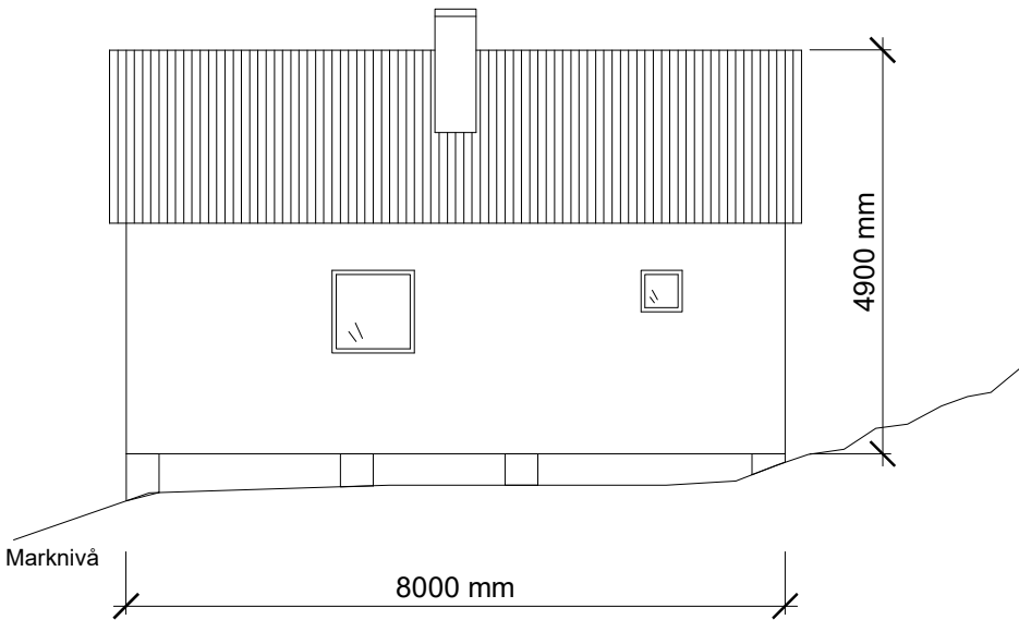
Fasad mot Sydöst
