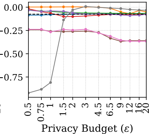
GitHub
