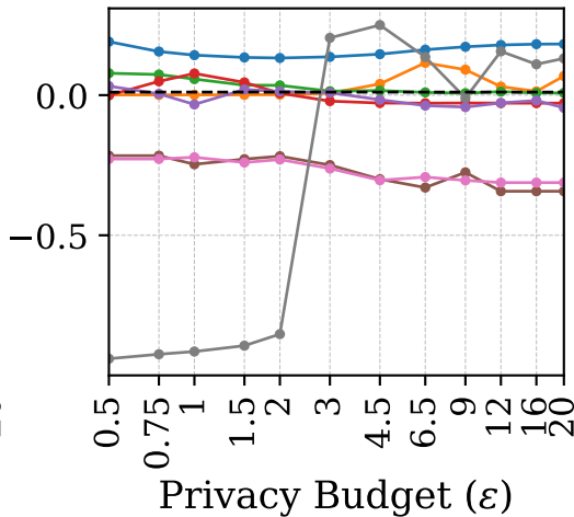
Brightkite
