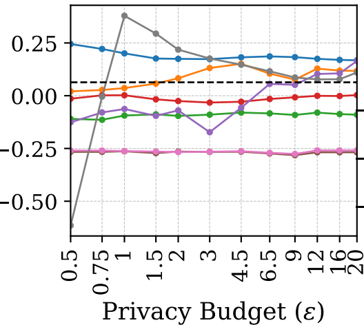
Facebook
