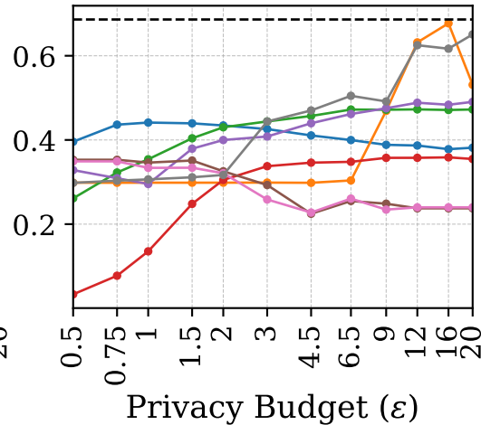
Brightkite
