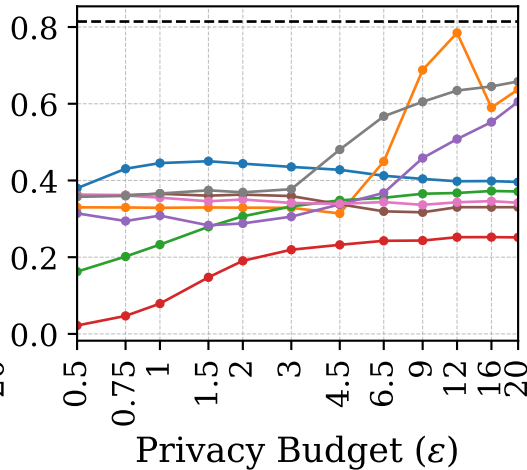
LastFM
