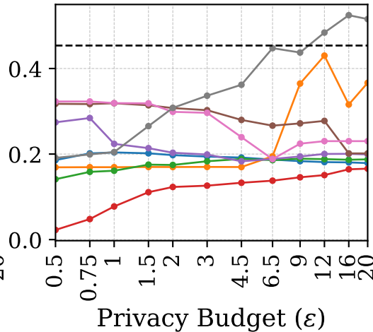
GitHub
