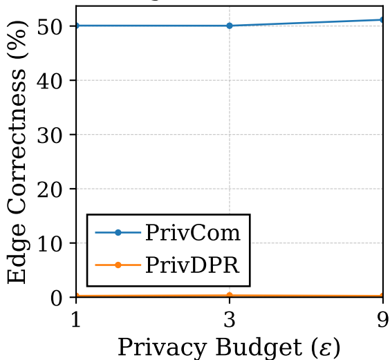
Edge Correctness
