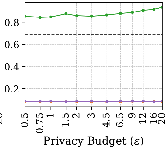
Brightkite
