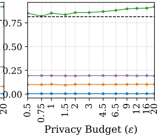
LastFM
