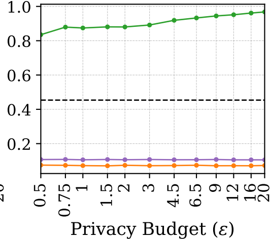
GitHub
