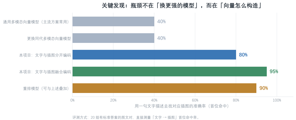
图 3 跨模态检索（文字到插图）准确率对比
