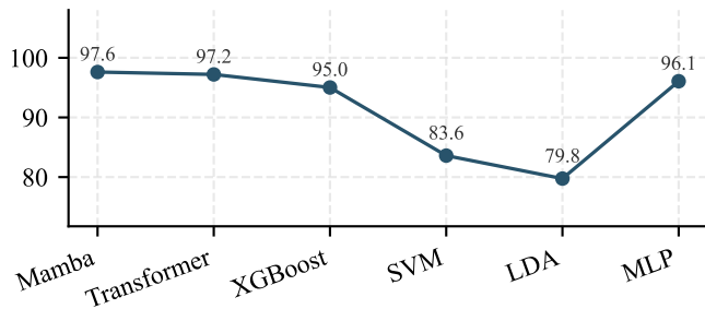
Precision
