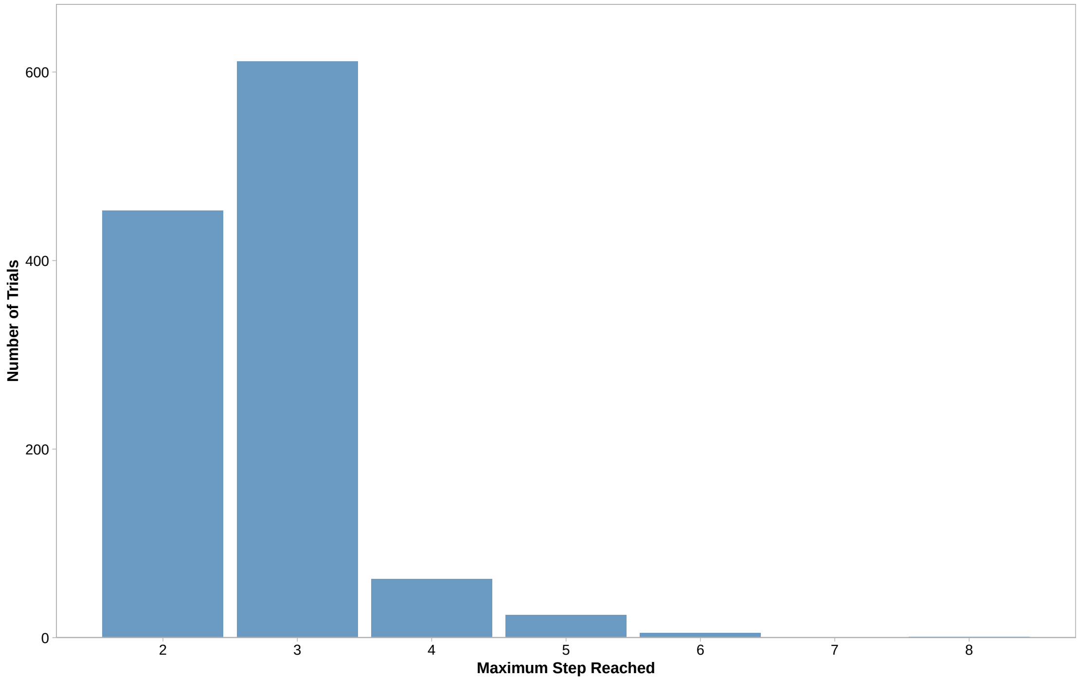
GPT-4.1 Mini
