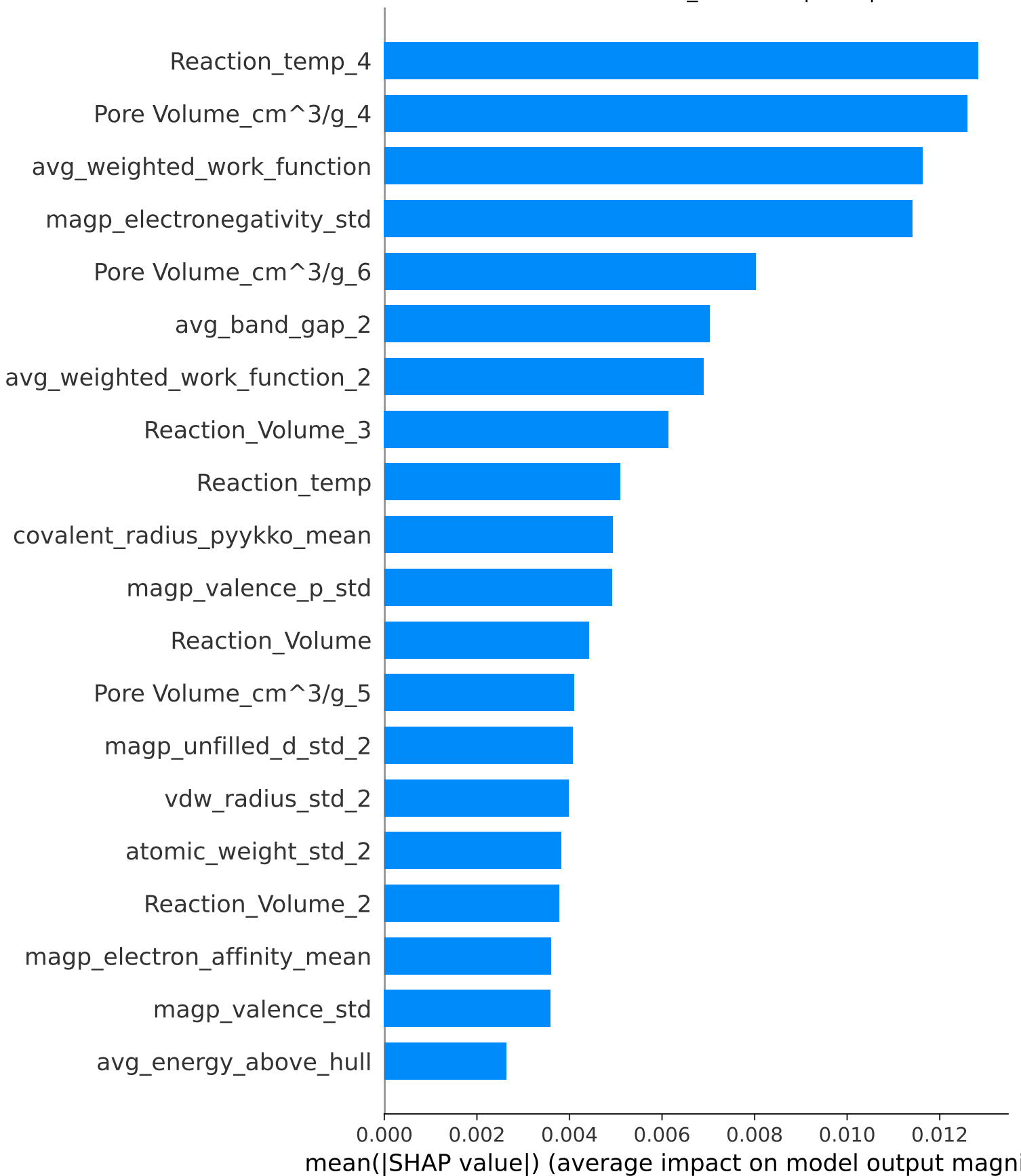
PRIDMO RF - mi_clf: Mean |SHAP|
