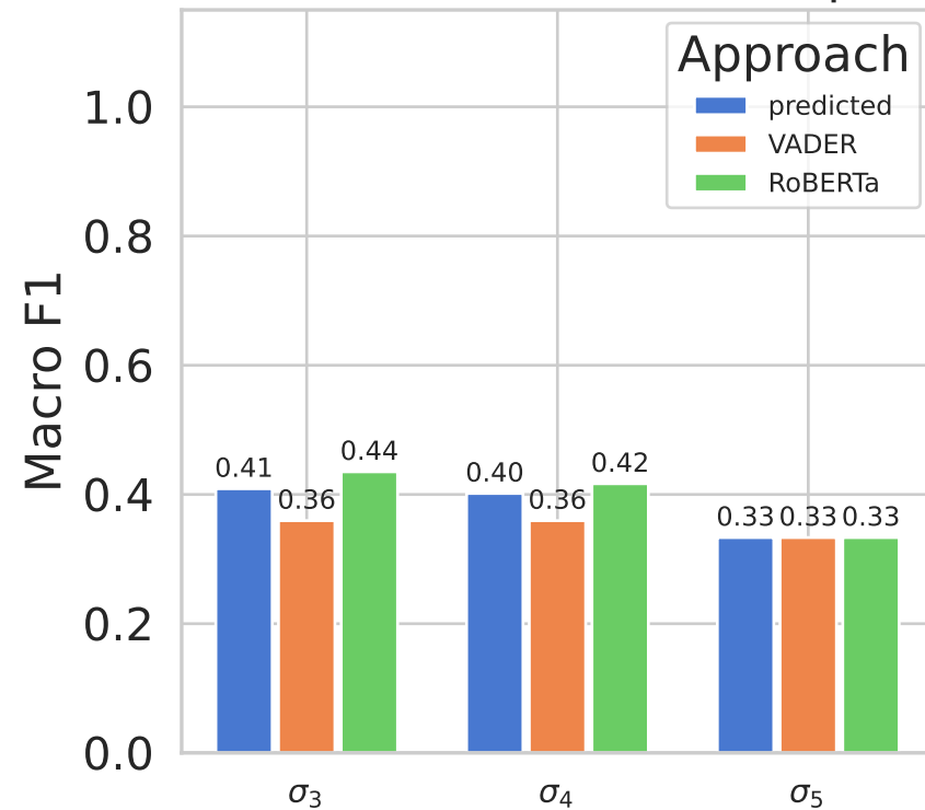
Macro F1 vs. Human GT (p3)
