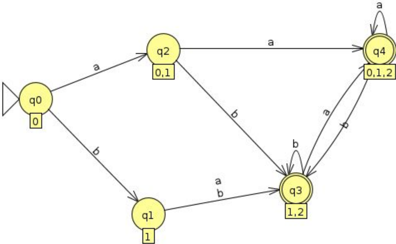
DFA
