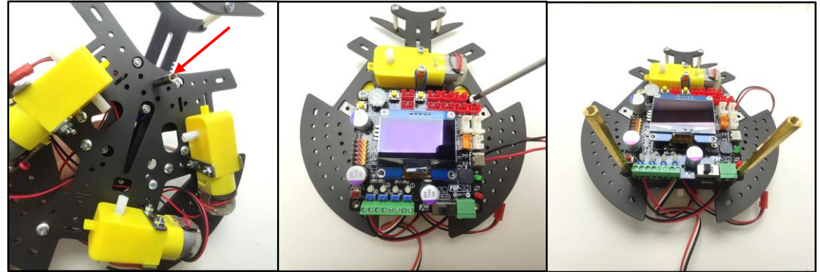
3.2 ชั้นเสารองโลหะขนาด 20 มม. เพื่อติดตั้งชุดยิงเข้ากับตัวหุ่นยนต์ ชั้นสกรู 3x6 มม. และเสารองยาว 60 มม. เพื่อยึด POP-32
