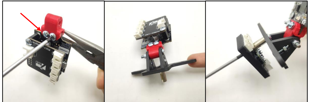
2.3 ใช้สกรู 3x15 มม. ยึดโมดูลกล้อง Pixy กับแขนยึด (ชิ้นส่วนสีแดง) ต่อมาให้นำแขนยึดไปติดตั้งเข้ากับแผ่นเสา โดยใช้สกรู 3x25 มม. และ น็อตตัวเมียกันคลาย สุดท้ายให้ติดตั้ง ZX-IMU กับเสารองโลหะด้านล่าง
