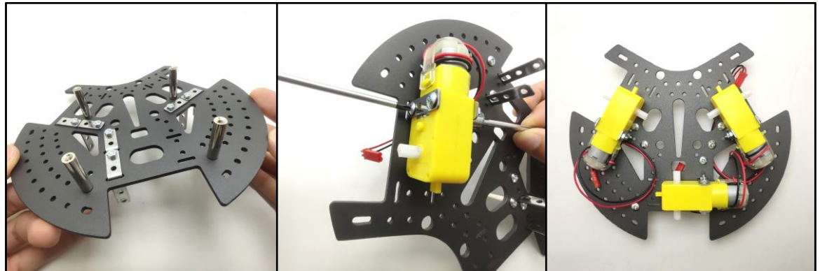
1.3 ติดตั้งเสาธงโลหะขนาด 25 มม. จำนวน 4 ตัว และใช้สกรู 3x25 มม. จำนวน 6 ตัวเพื่อติดตั้งมอเตอร์ BO1 เข้ากับฉากโลหะ
