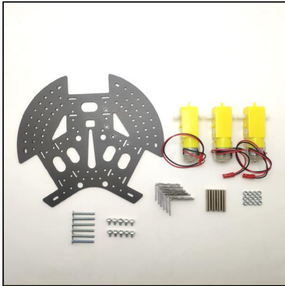
1.1 เตรียมอุปกรณ์ดังนี้
