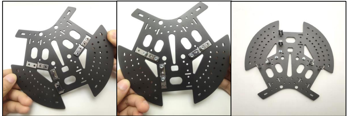
1.2 ใช้สกรู 3x6 มม. จำนวน 6 ตัว ร้อยผ่านแผ่นฐาน ฉากโลหะ ขนาด 2x3 จำนวน 3 ตัว และขันให้แน่นด้วยน็อตตัวเมีย
