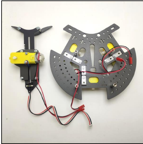
3.1 เตรียมตัวหุ่นยนต์และชุดยิง
