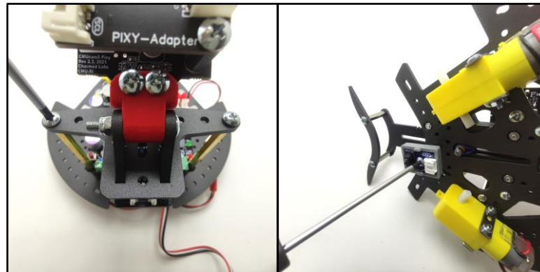
3.3 ใช้สกรู 3x6 มม. จำนวน 2 ตัว เพื่อยึดฐานเซนเซอร์เข้ากับตัวหุ่นยนต์ และใช้สกรู 3x8 มม. เพื่อยึดเซนเซอร์ ZX-03
