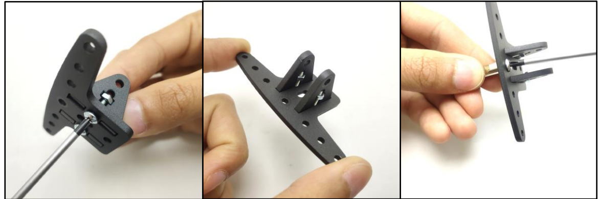
2.2 ประกอบแผ่นเสากับแผ่นฐานเข้าด้วยกัน ด้วยสกรู 3x12 มม. จำนวน 2 ตัว และเสารองโลหะยาว 15 มม. ด้วยสกรู 3x6 มม.
