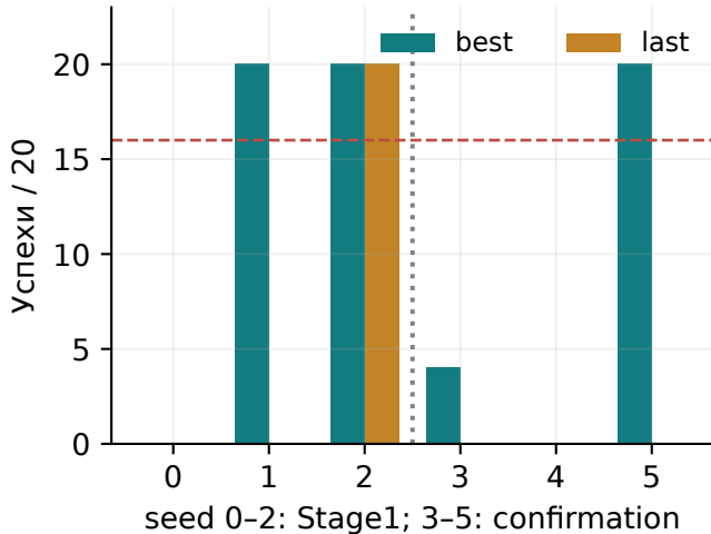
DDPG-on · warmup5000
