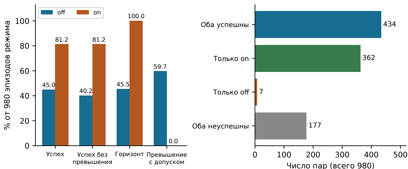
Рисунок 9 – Слева — отдельные метрики по 980 эпизодам каждого режима; справа — взаимоисключающие исходы 980 пар. Части слева пересекаются и не должны суммироваться до 100%.
