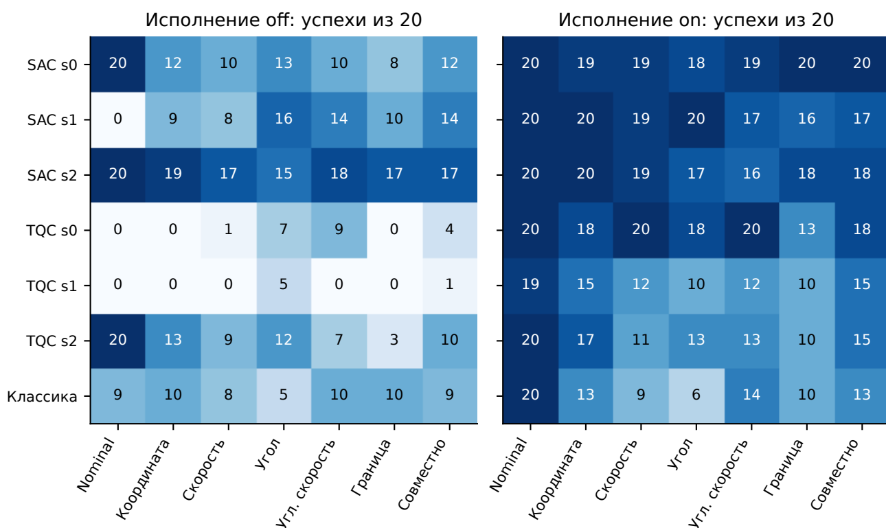
Рисунок 8 – Полная матрица успеха фиксированных контроллеров: каждое число из 20 общих состояний группы. Off/on — исполнение одних весов. Таблица цветов дополнена числами для чтения в чёрно-белой печати.
