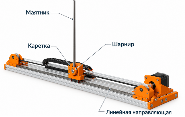
Рисунок 2 – Основные узлы установки. Иллюстрация, созданная с помощью ИИ; не фотография и не точный технический чертёж.
