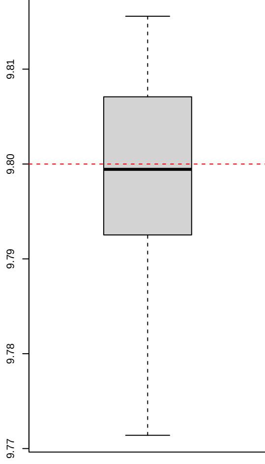
Posterior mean of g
