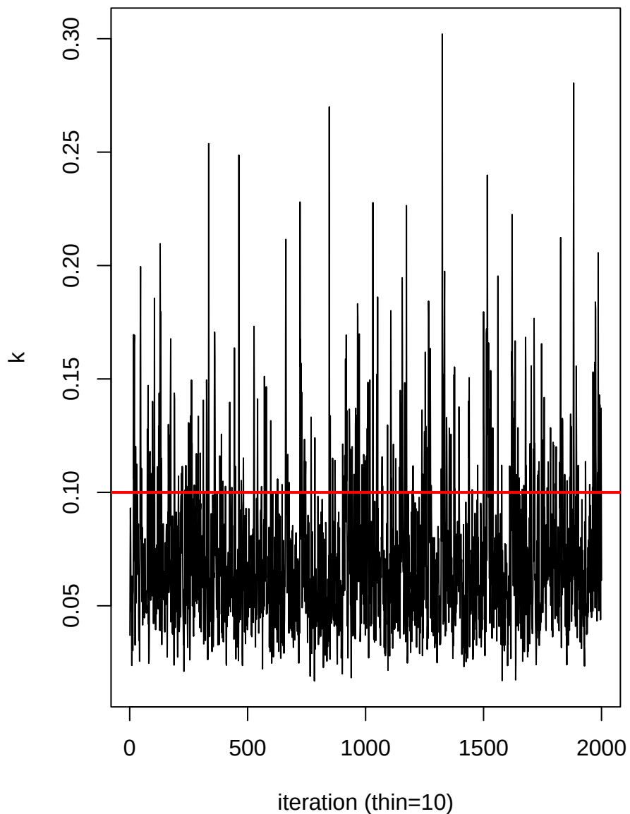
Trace plot: k
