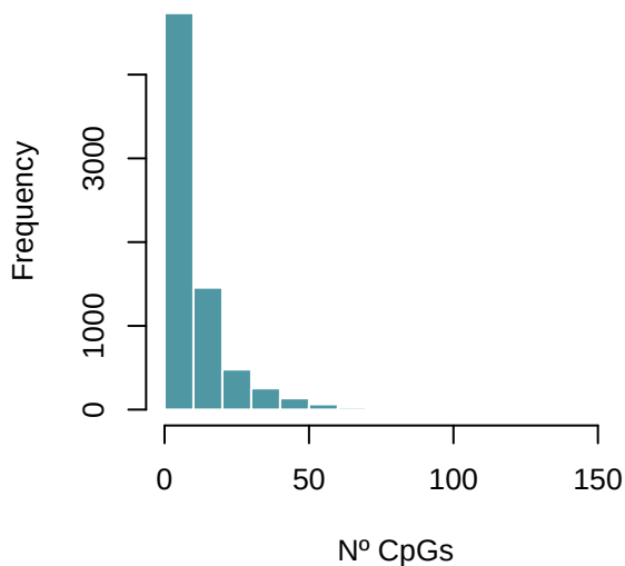
CpGs per DMR
