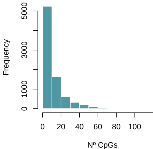
CpGs per DMR
