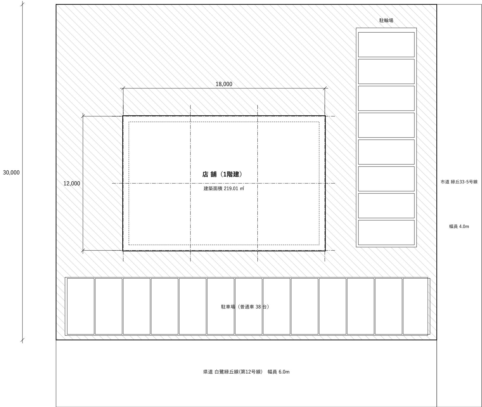
配置図 S=1/200
