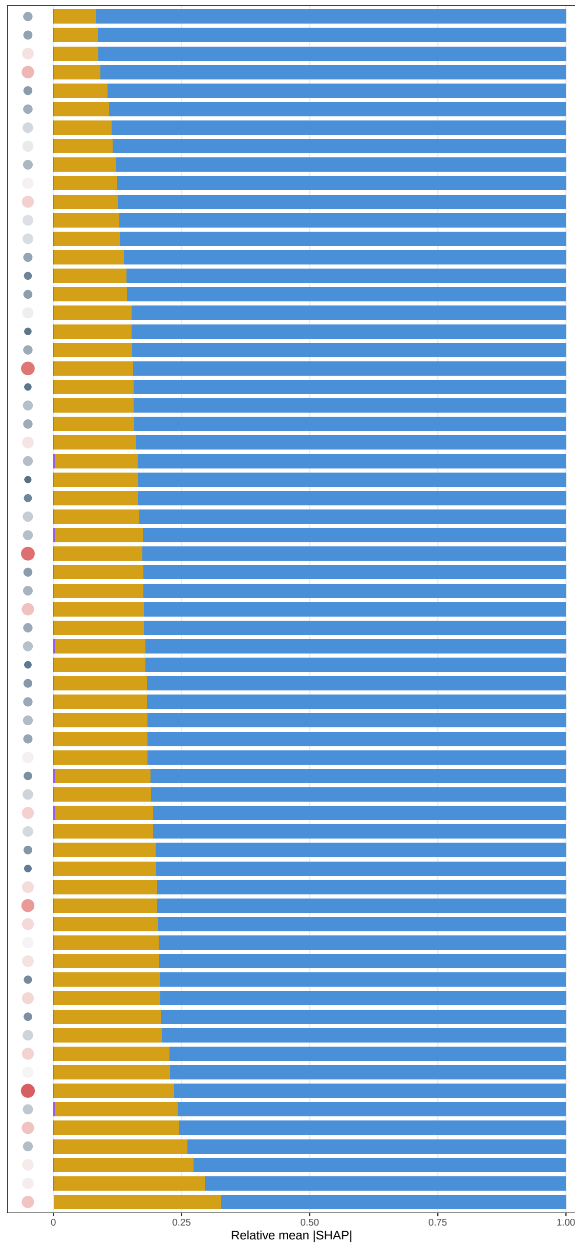
M6 anom (C+T+D+Mem) | 24m window | WUE (g C mm... 3 )
