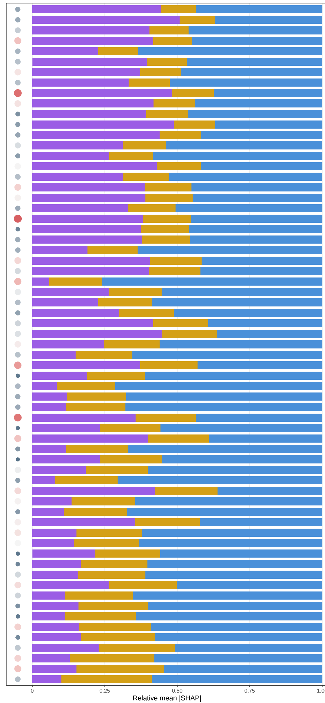
M6 raw (C+T+D+Mem) | 12m window | ETmax (mm d... 1 )
