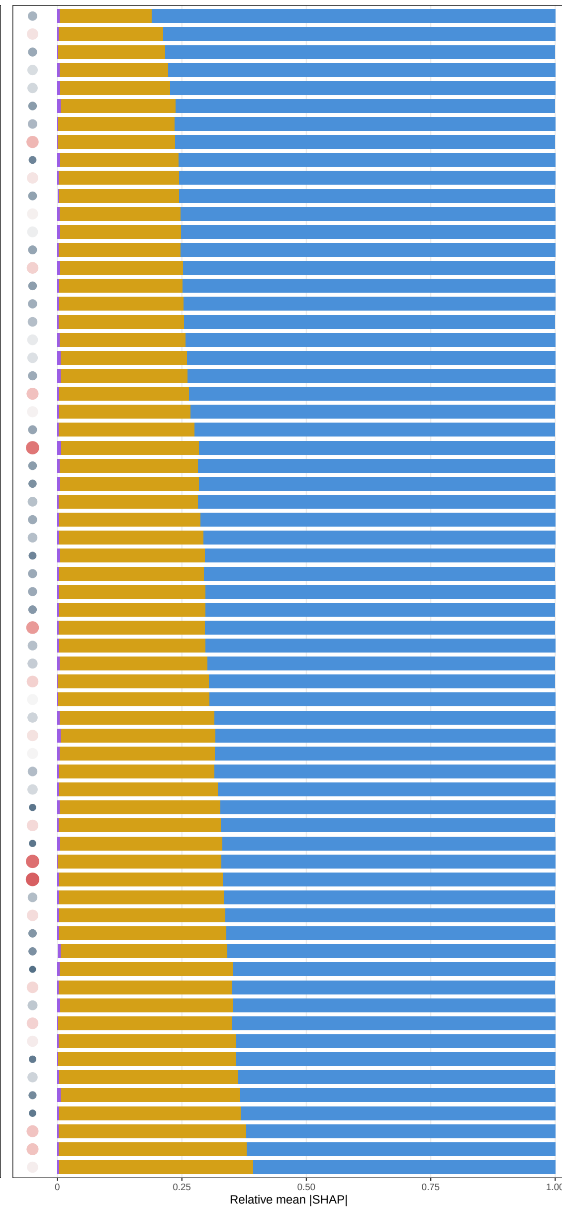
M6 anom (C+T+D+Mem) | 12m window | uWUE (g C mm... 1
