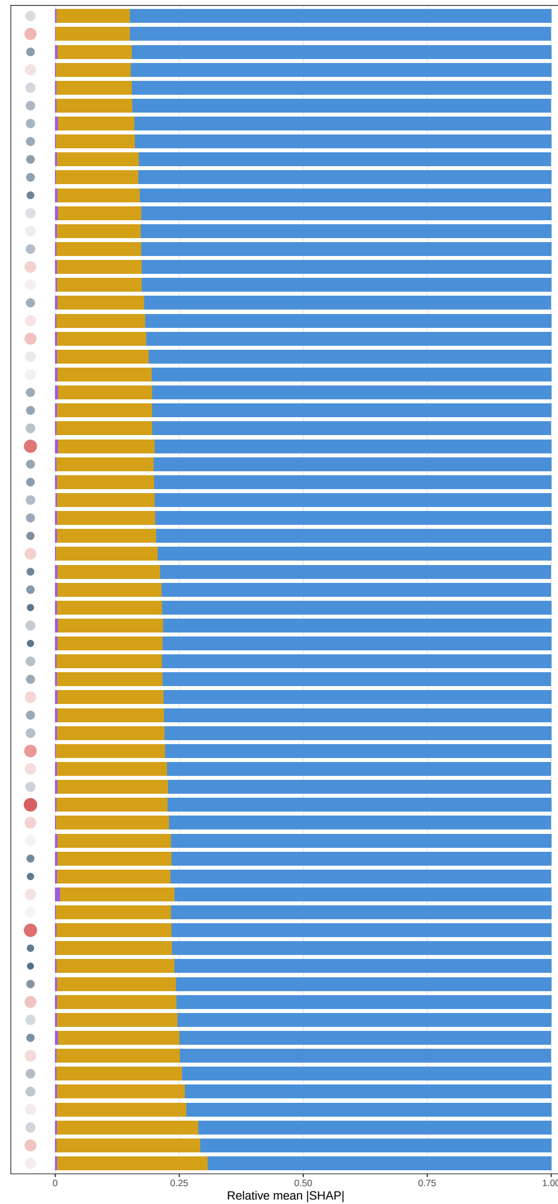
M6 anom (C+T+D+Mem) | 24m window | uWUE (g C mm... 1
