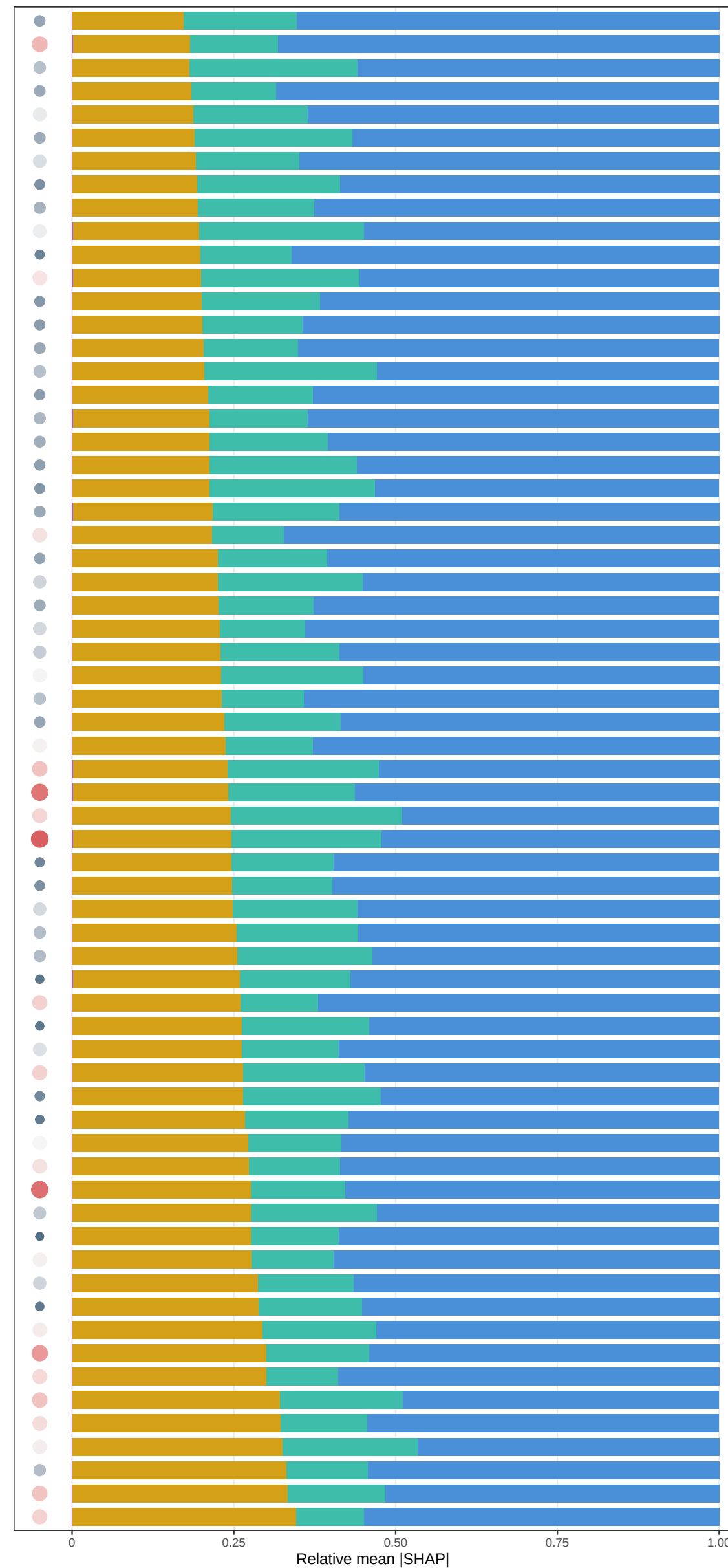
M8 anom (C+T+D+Mem) | 12m window | WUE (g C mm... -1 )
