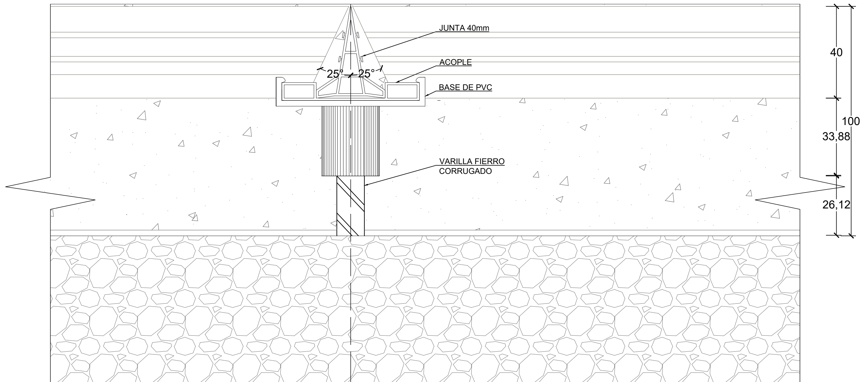
DETALLE DE INTERSECCIÓN JUNTAS 40mm Esc. 1:1
