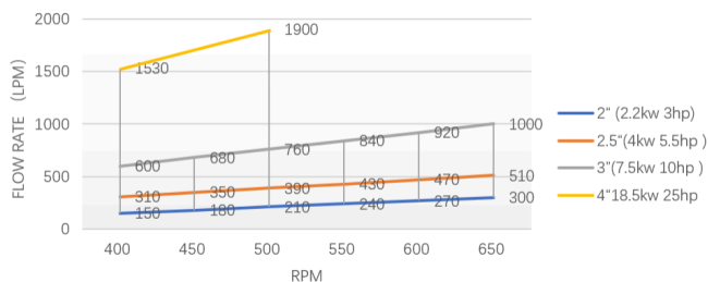
Curva de Flujo vs RPM
