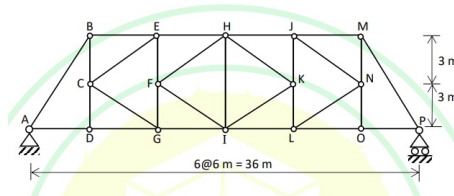
Fig. 1.2.8.1. Pin-jointed truss for Q14.
