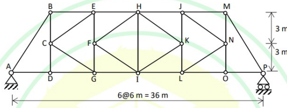
Fig. 3. Pin-jointed truss for Q14.
