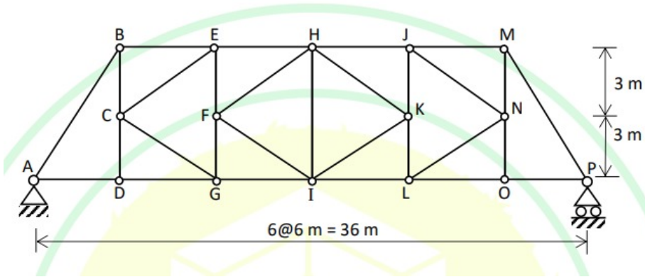
Fig. 1.2.8.1. Pin-jointed truss for Q14.
