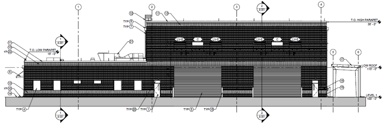
1 SOUTH ELEVATION A-202 SCALE: 1/8" = 1'-0"
