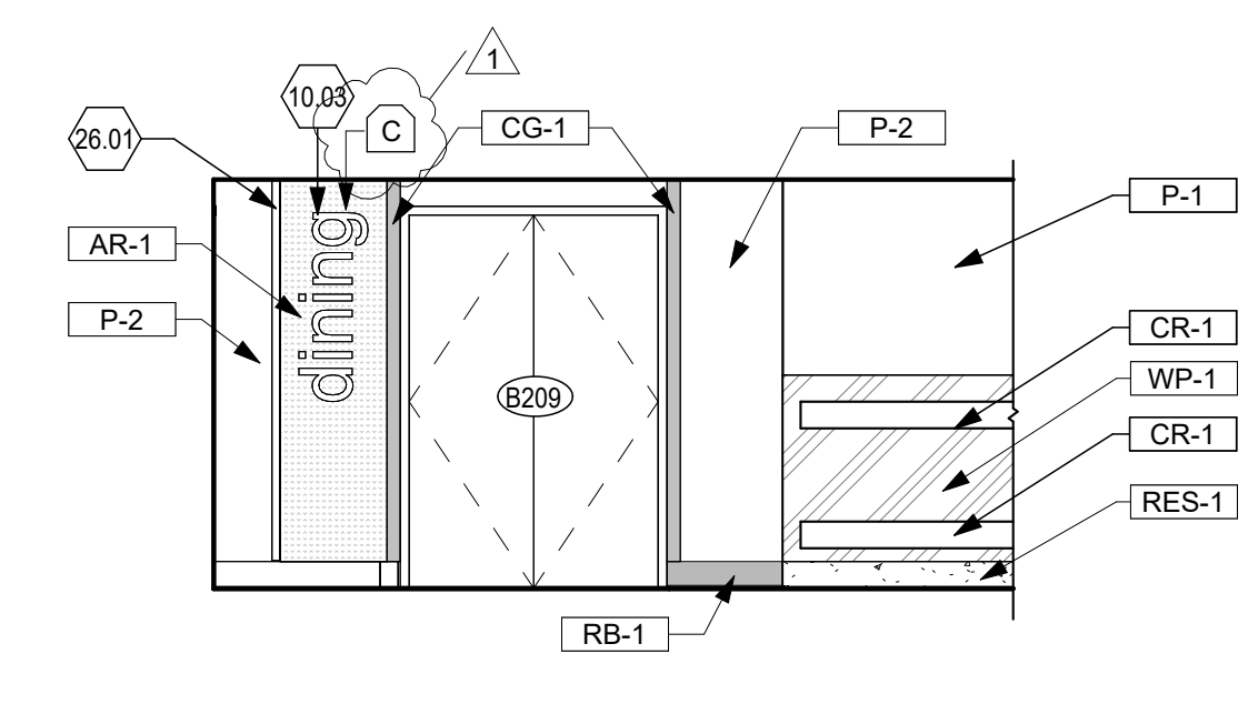
7 B209 Scale: 1/4" = 1'-0"
