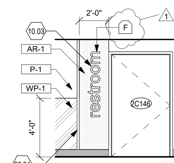
15 2C146 Scale: 1/4" = 1'-0"
