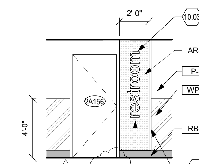
13 2A156 Scale: 1/4" = 1'-0"
