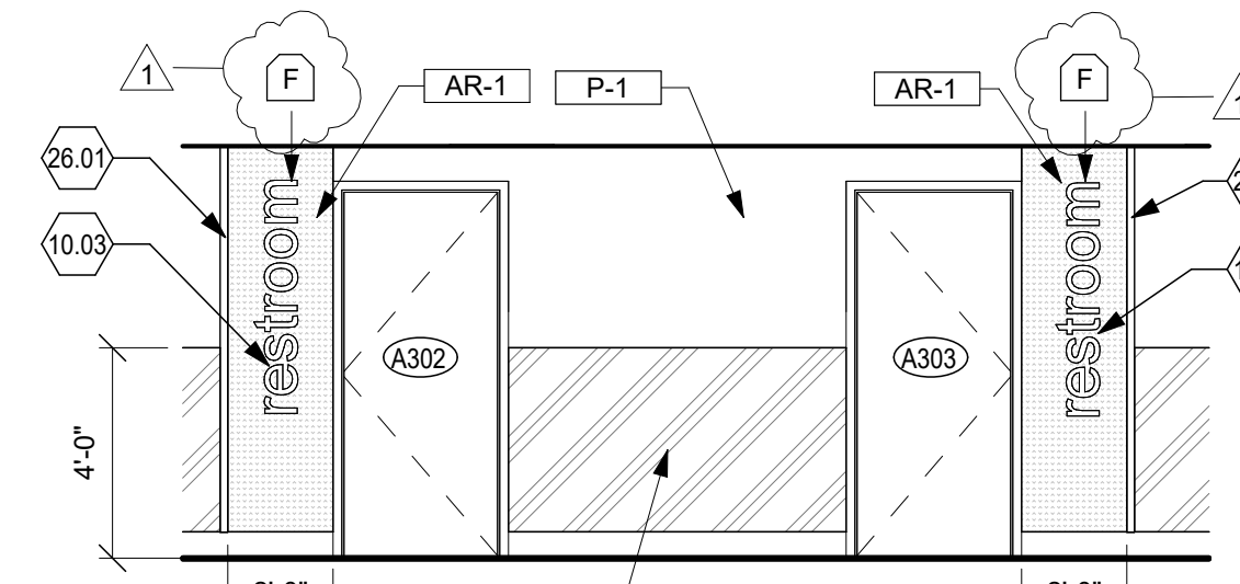
14 A302 Scale: 1/4" = 1'-0"
