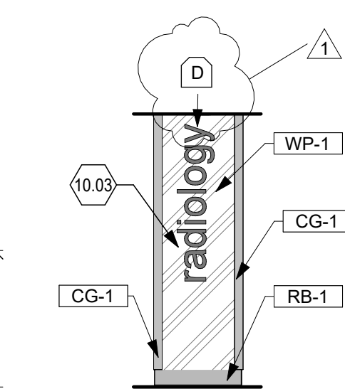
10 D312A - NORTH Scale: 1/4" = 1'-0"
