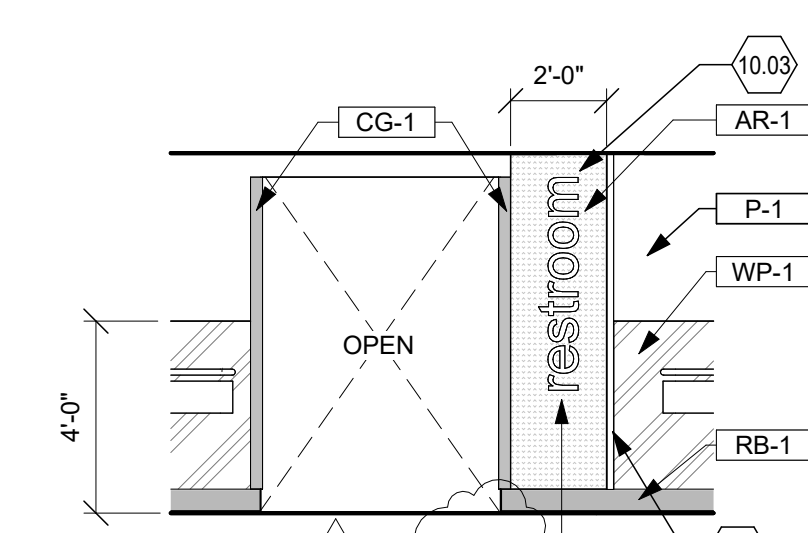
12 B201 & B202 Scale: 1/4" = 1'-0"
