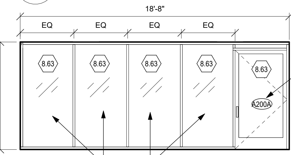
4 A200 Scale: 1/4" = 1'-0"
