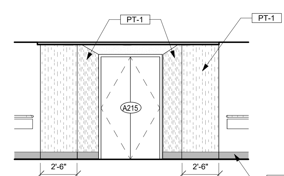
17 A215 Scale: 1/4" = 1'-0"
